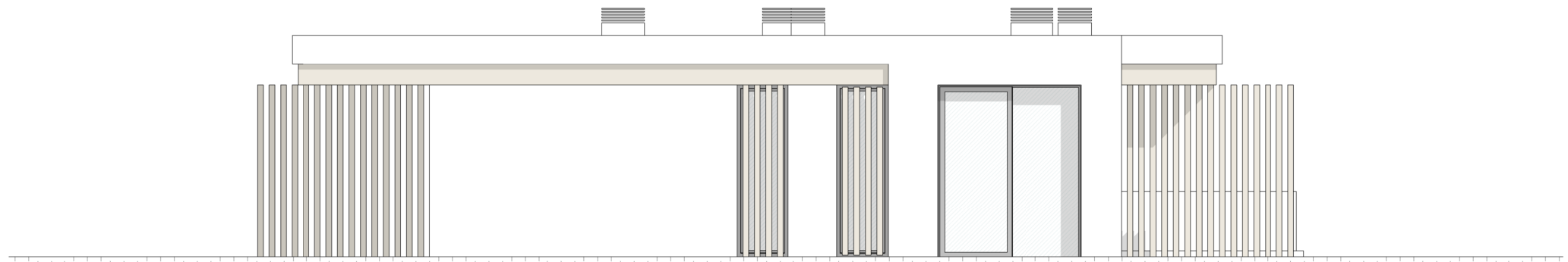
Alçado Nascente
