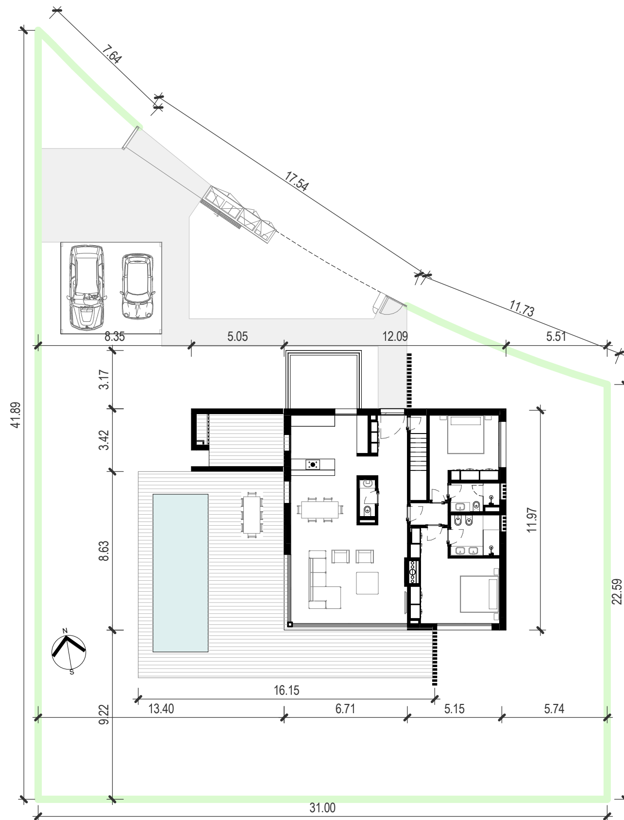
PLANTA DE IMPLANTAÇÃO M64
