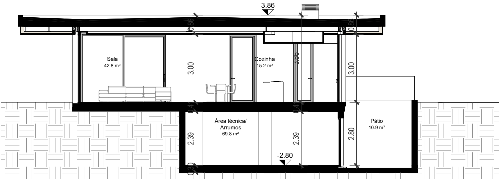
Corte Longitudinal 1 : 100
